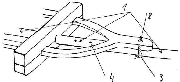
5. Teilstück vom Hintergestell des Ackerwagens.
